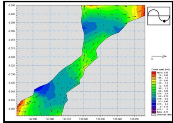
Gambar 10. Vektor kecepatan arus pada saat surut
