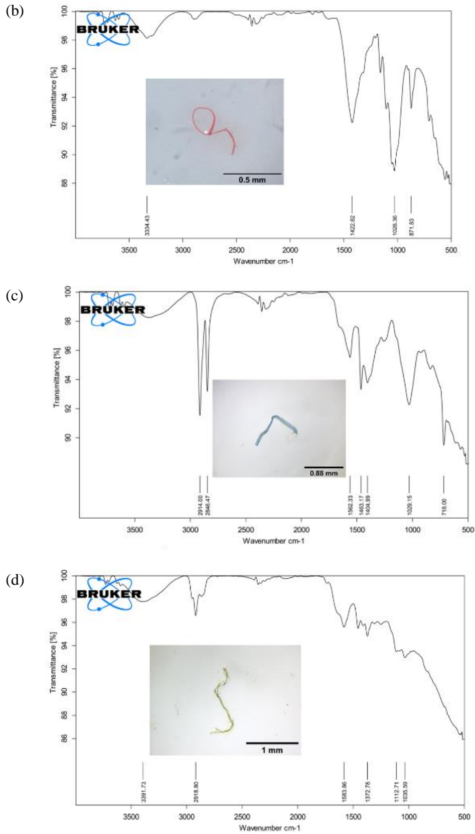
Gambar 5. Hasil spektrum FTIR pada empat jenis partikel mikroplastik. (a) Polyester (PES), (b) Polypropylene (PP), (c) Polyethylene (PE), (d) Polyurethane (PU).
