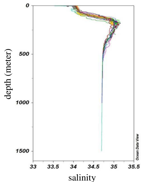
Gambar 2. Profil vertikal salinitas terhadap kedalaman.
