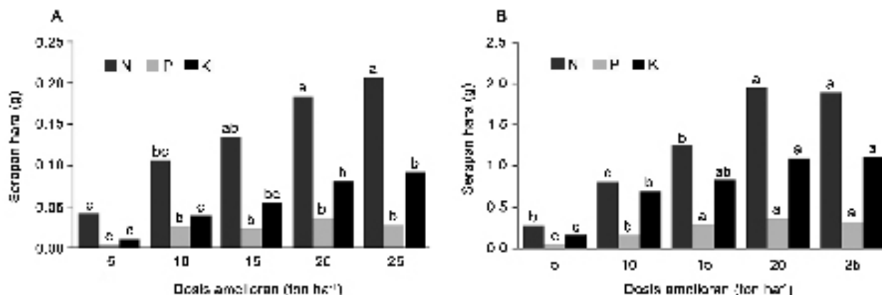
Gambar 3. Pengaruh dosis amelioran terhadap serapan NPK oleh akar (A) dan tajuk (B). Keterangan: huruf yang sama pada unsur yang sama menunjukkan tidak berbeda nyata berdasarkan uji DMRT \alpha = 5\%
