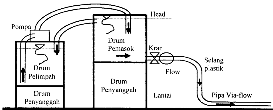
Gambar 1. Skema peralatan percobaan pada head 1,8 m
