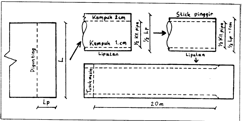
Gambar 5. Skema pembuatan pipa pipih tipe B
