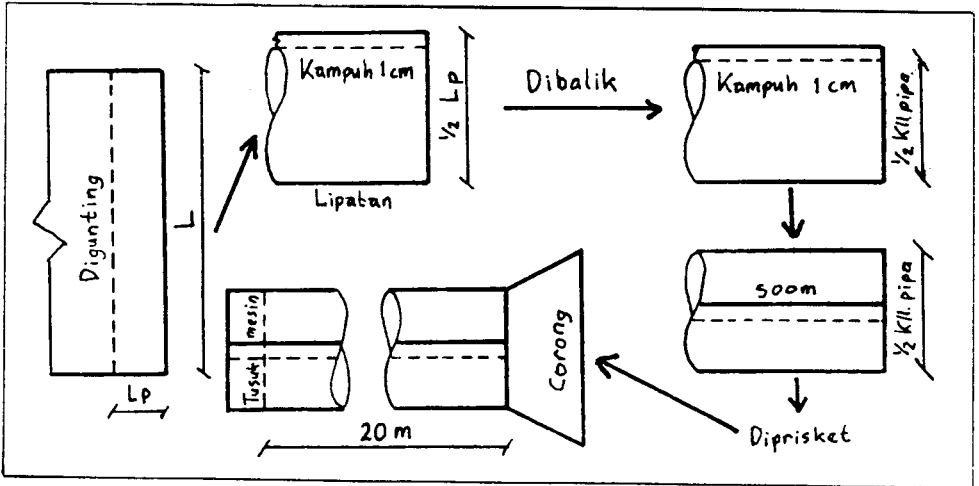
Gambar 4. Skema pembuatan pipa pipih tipe A
