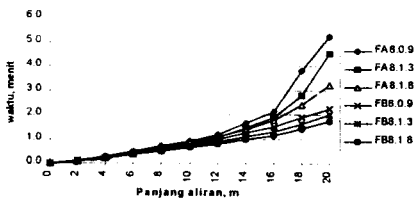
Gambar 2. Kurva kecepatan aliran pada pipa Famatex dengan keliling 8 cm
