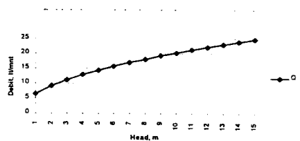
Gambar 3. Kurva hubungan debit keluar pada berbagai tekanan operasional
