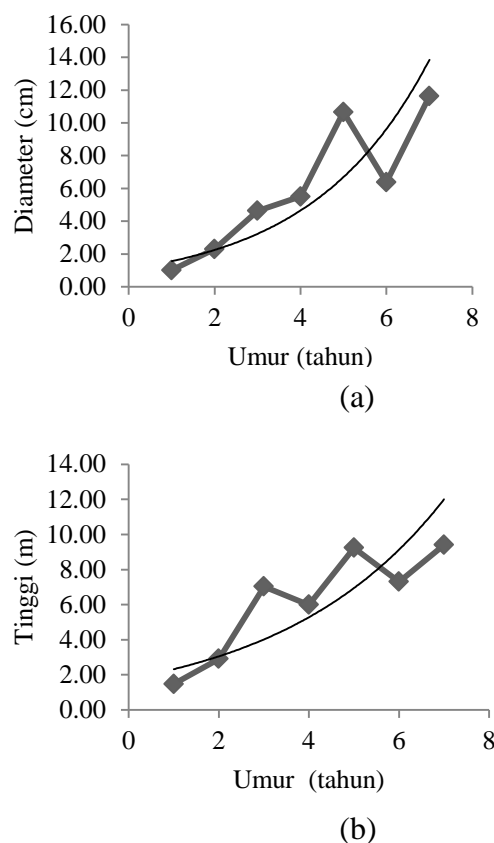
Gambar 1 Kurva pertumbuhan S. leprosula : (a) diameter; (b) tinggi
