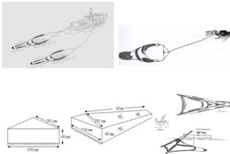
Gambar 4 Kelompok trawl, garuk dan pukat dorong
