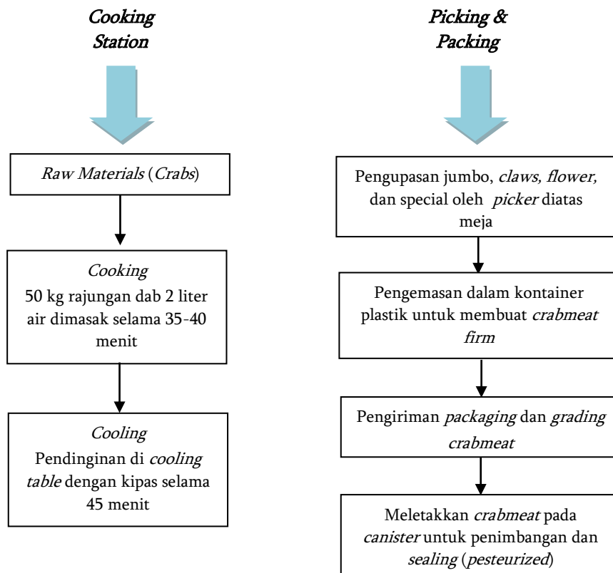
Gambar 3 Skema pengolahan rajungan di cooking staton dan miniplant
