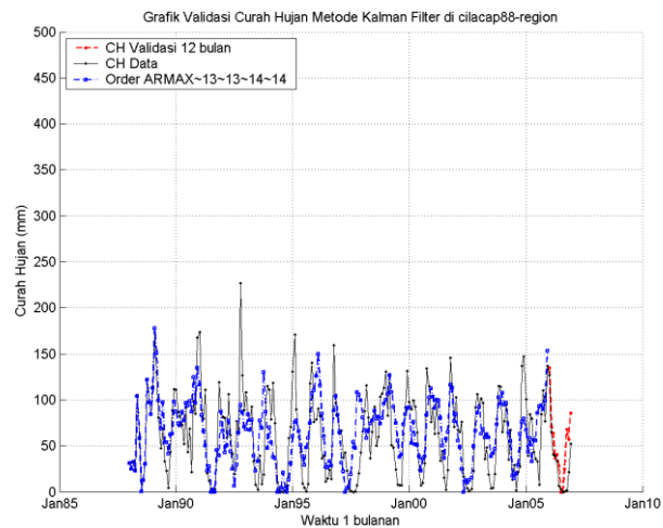
Gambar 8. Fluktuasi curah hujan antara data pengamatan dan hasil simulasi selama periode 1988-2006
