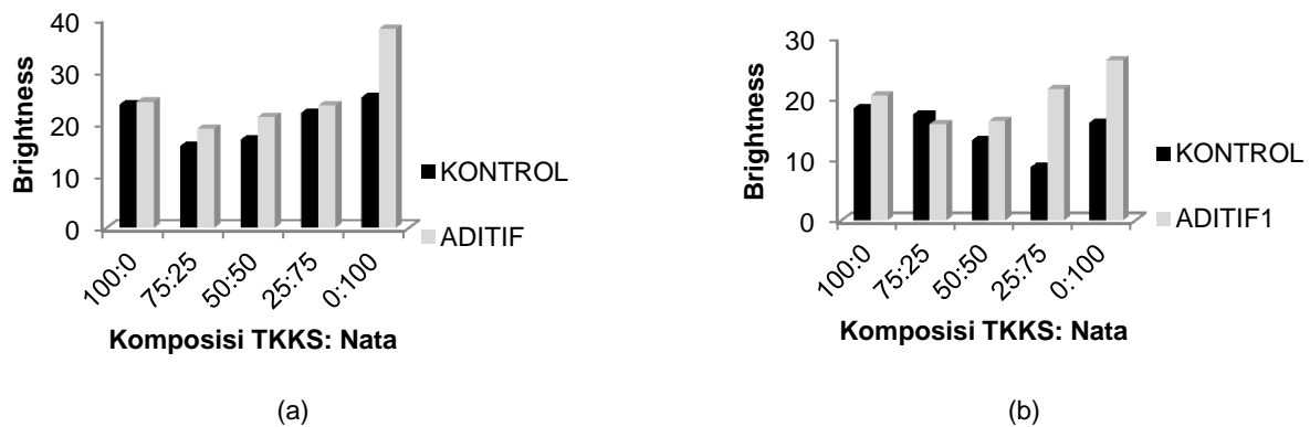
Gambar 8 (a) Derajat putih untuk gramatur target 60 g/m 2 ; (b) Derajat putih untuk gramatur target 120 g/m 2 .
