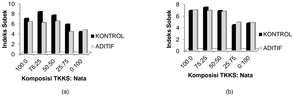
Gambar 5 (a) Indeks sobek untuk gramatur target 60 g/m 2 ; (b) Indeks sobek untuk gramatur target 120 g/m 2 .
