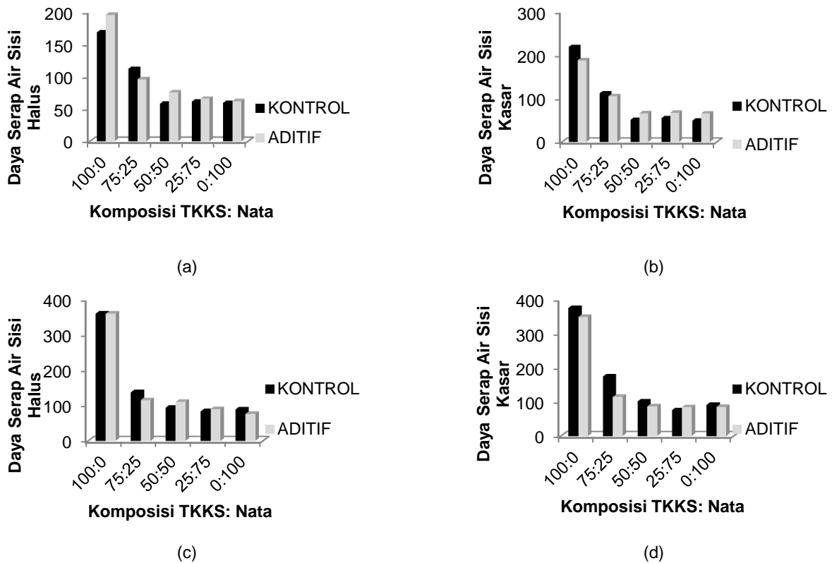
Gambar 7 (a) Daya serap air sisi halus untuk gramatur target 60 g/m 2 ; (b) Daya serap air sisi kasar untuk gramatur target 60 g/m 2 ; (c) Daya serap air sisi halus untuk gramatur target 120 g/m 2 ; (d) Daya serap air sisi kasar untuk gramatur target 120 g/m 2 .
