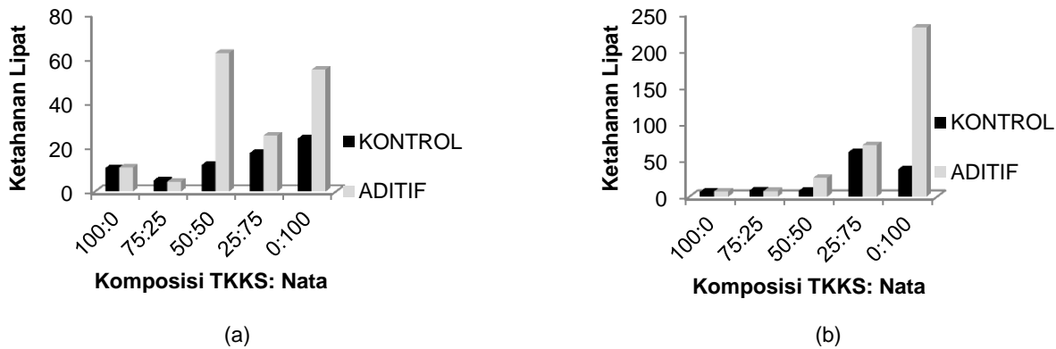
Gambar 6 (a) Ketahanan lipat untuk gramatur target 60 g/m 2 ; (b) Ketahanan lipat untuk gramatur target 120 g/m 2 .
