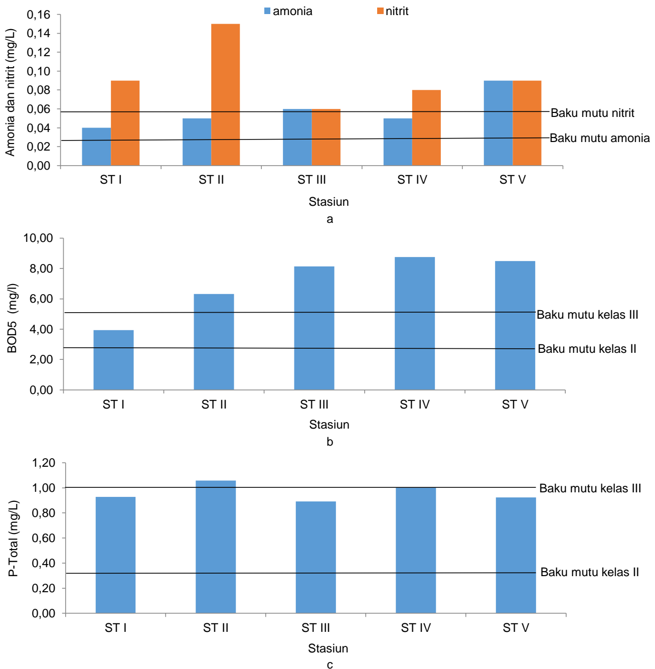
Gambar 3 Nilai rata-rata konsentrasi parameter yang telah melebihi baku mutu air Kelas II dan III (a: amonia dan nitrit, b: BOD 5 , dan c: P-total).
